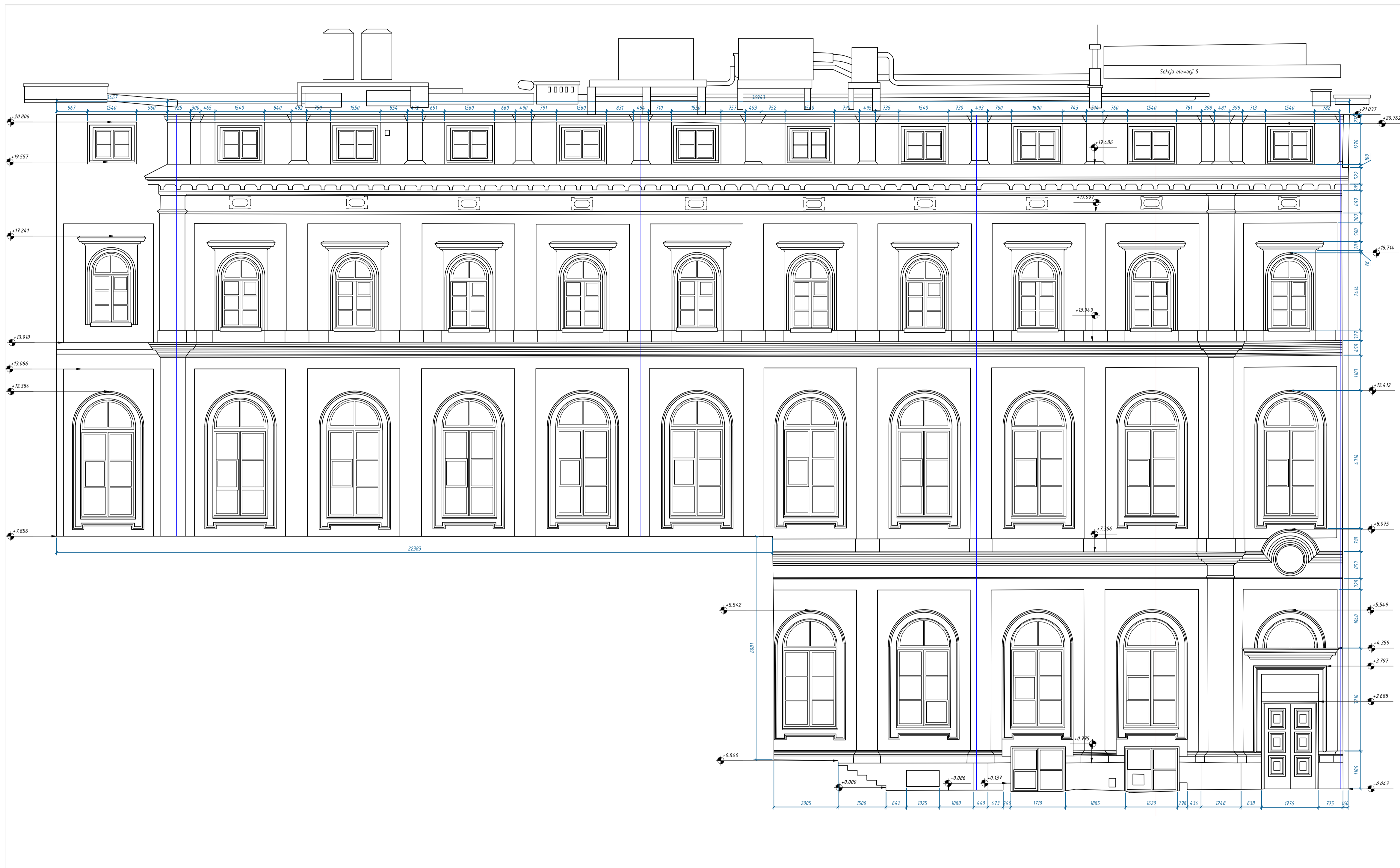
Elewacja 5 (1 : 50)
